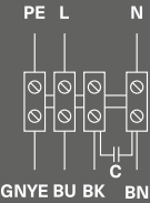
Схема 1 (230 В, 1 ф, 50 Гц.)
