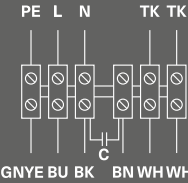
Схема 2 (230 В, 1 ф, 50 Гц.)
