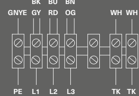
Схема 2 (400 В, 3 ф, 50 Гц.)
