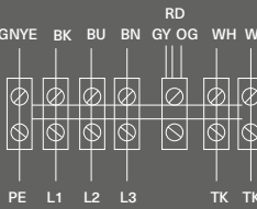
Схема 2 (400 В, 3 ф, 50 Гц.)
