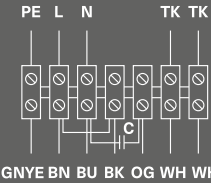
Схема 3 (400 В, 3 ф, 50 Гц.)
