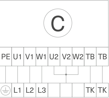
Схема 2 (3 ~ 400 В)
