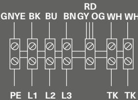
Схема 4 (Δ — 400 В, 3 ф.)
