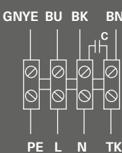
Схема 3 (△ — 230 В, 3 ф.)
