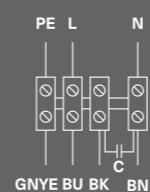
Схема 1 (230 В, 1 ф, 50 Гц.)
