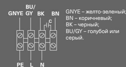
Схема 1 (230 В, 1 ф.)
