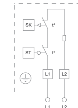
Схема 2 (400 В, 2 фазы)
