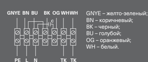
Схема 2 (230 В, 1 ф.)
