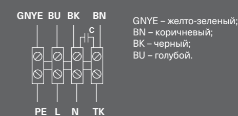
Схема 3 (△ — 230 В, 3 ф.)
