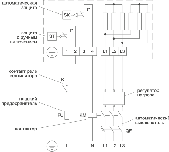
9, 12 кВт
