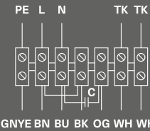
Схема 3 (400 В, 3 ф, 50 Гц.)
