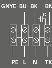
Схема 3 (△ — 230 В, 3 ф.)
