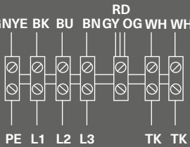
Схема 4 (λ — 400 В, 3 ф.)
