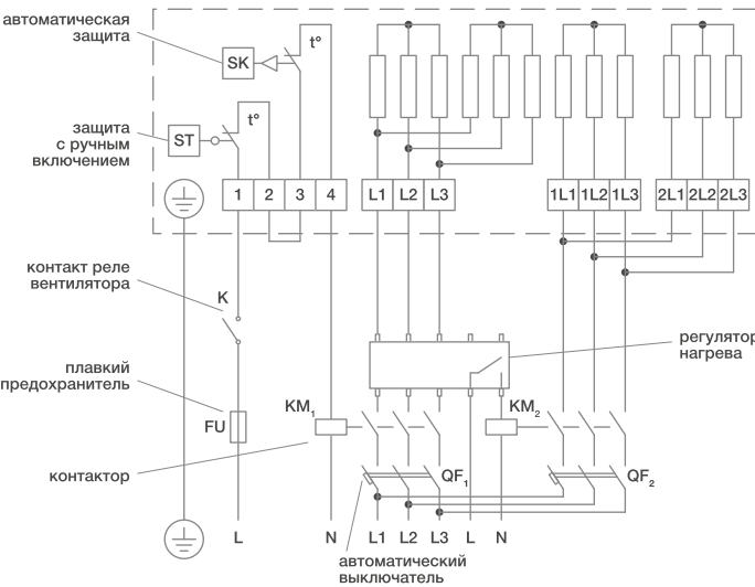
30 кВт
