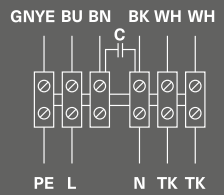
Схема 1 (230 В, 1 ф, 50 Гц.)
