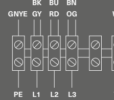
Схема 2 (400 В, 3 ф, 50 Гц.)
