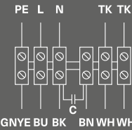
Схема 2 (230 В, 1 ф, 50 Гц.)
